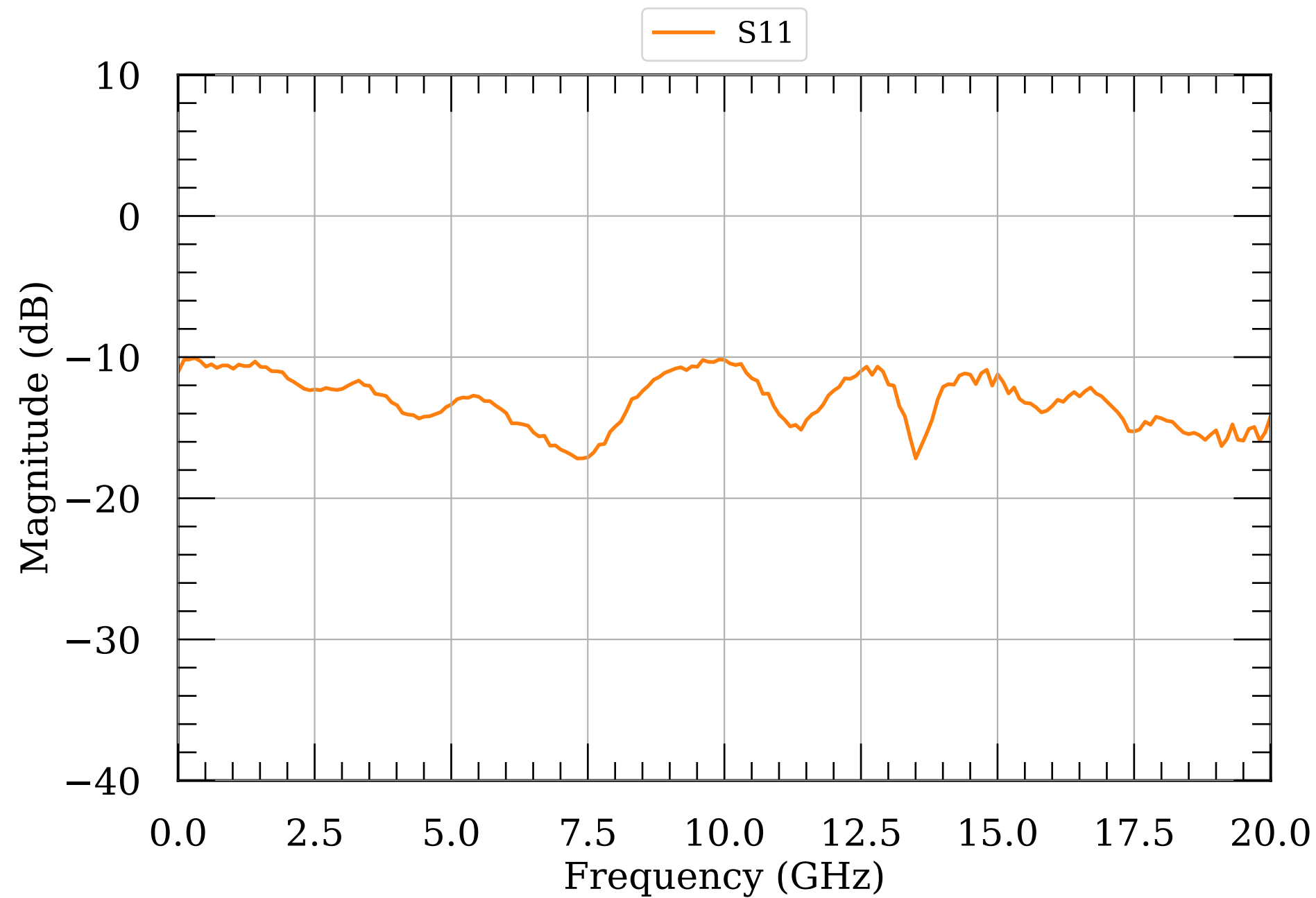
LNA S-params module064
